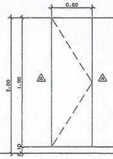
② บานประตูห้องน้ำผ้าแดงรูป เกล็ดปลาใบพัด กระจกนิรภัย กระจกนิรภัย 2"x4"
