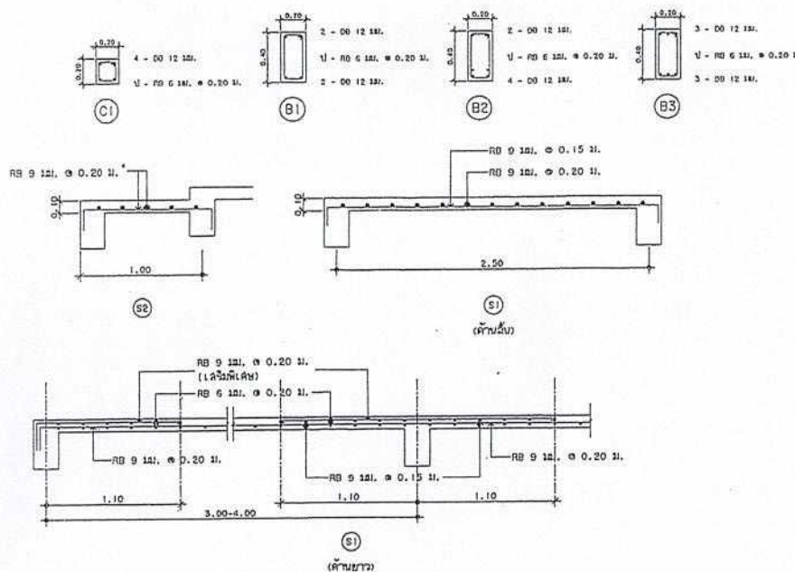
แปลนโครงสร้างหลังคาห้องน้ำ มาตราส่วน 1:50 แบบปรับปรุงรายการที่ (10)
