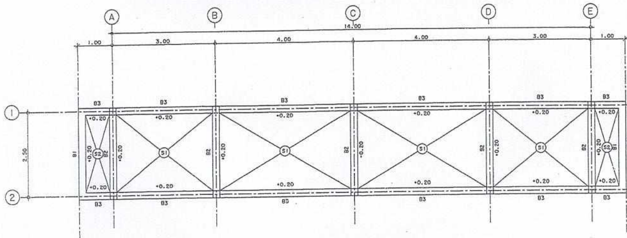
แปลนคานาพื้นห้องน้ำหญิง ภาคขวาง 1:50 (แบบปรับปรุงรายการที่ (11))
