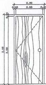
① ชุดประตูบานเปิด PVC, ฉายไม้ รูปทรงคานประตู วงกบไม้เนื้อแข็ง 2"x4"
