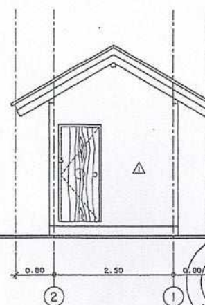
รูปด้านขวาห้องน้ำหญิง ภาคเช้า 1:50 (แบบปรับปรุงรายการที่ 11)
