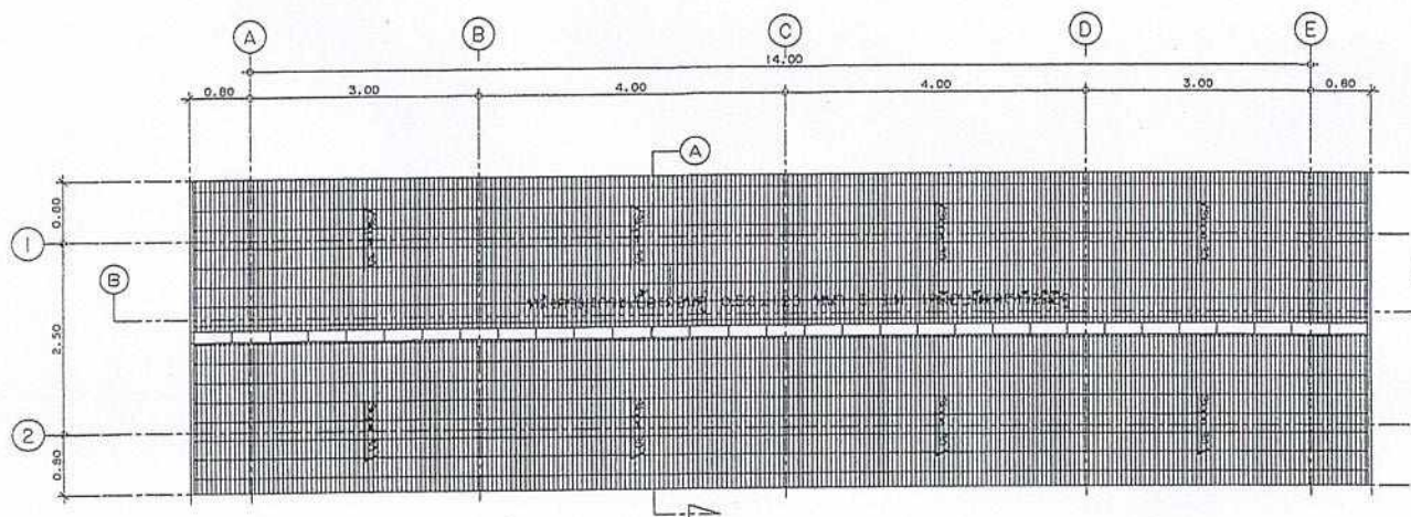
แผนผังห้องน้ำชาย (ก่อสร้างใหม่นอกอาคาร)
