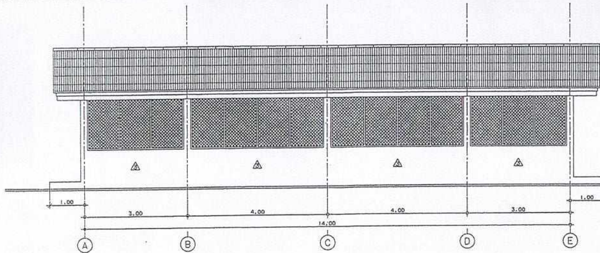
รูปด้านหน้าห้องน้ำชาย มาตราส่วน 1:50 (แบบรับปรุงรายการที่ 10)
