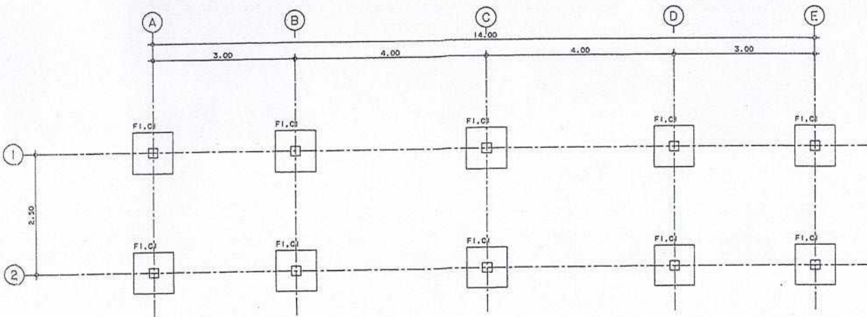
แปลนฐานจากห้องน้ำหญิง ภาคขวาง 1:50 (แบบปรับปรุงรายการที่ (11))
