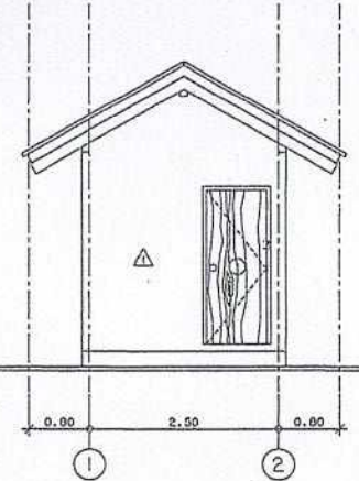
รูปด้านซ้ายห้องน้ำชาย มาตราส่วน 1:50 (แบบรับปรุงรายการที่ 10)
