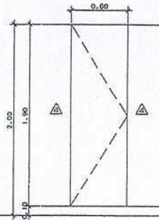
② บานประตูบานเปิด PVC, ฉายไม้ รูปทรงคานประตู วงกบไม้เนื้อแข็ง 2"x4"
