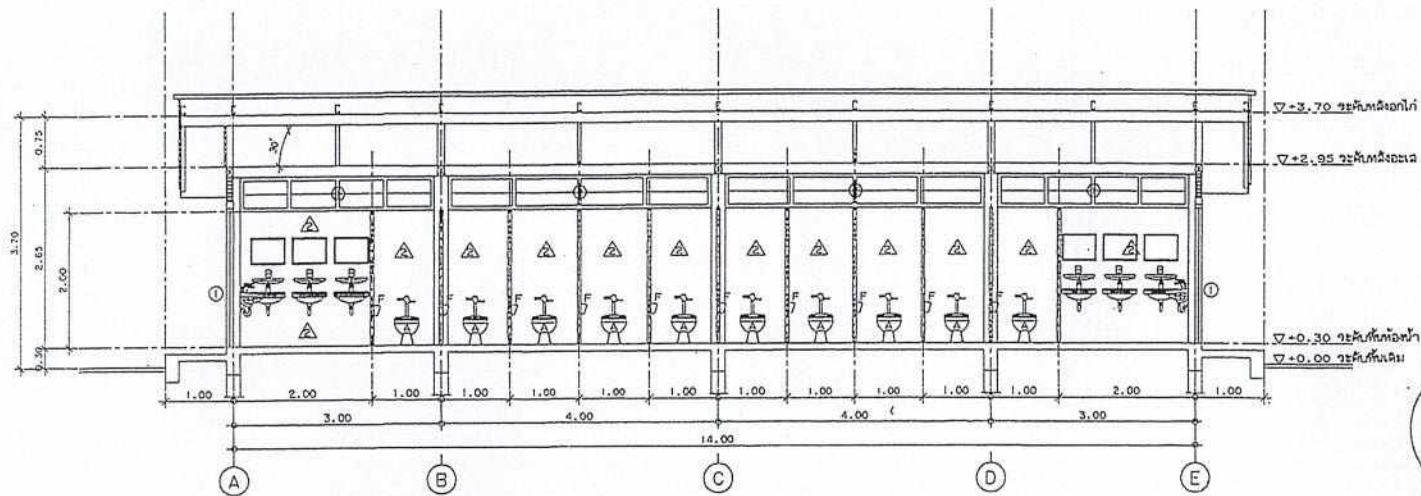
รูปตัด B ห้องน้ำหญิง มาตราส่วน 1:50 แบบปรับปรุงรายการที่ (11)
