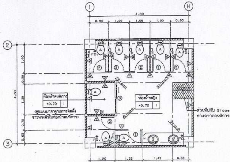
แปลนห้องน้ำดิบ ชั้นที่ 1 มาตราส่วน 1:50 (แบบปรับปรุงรายการที่ 2)
