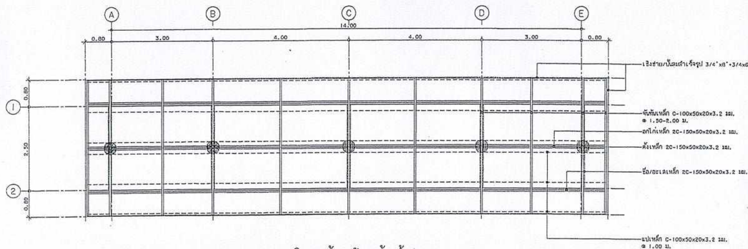
แปลนโครงสร้างหลังคาห้องน้ำ มาตราส่วน 1:50 แบบปรับปรุงรายการที่ (10)
