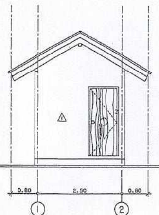
รูปด้านซ้ายห้องน้ำหญิง มหาดล้น 1:50 (แบบปรับปรุงรายการที่ 11)
