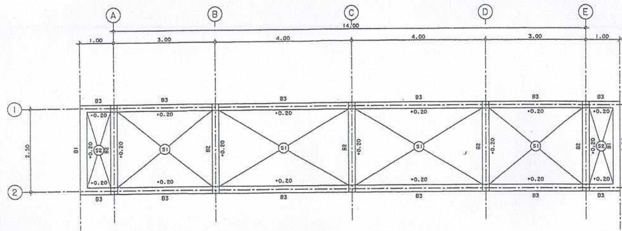
แปลนคานพื้นห้องน้ำชาย มาตราส่วน 1:50 (แบบรับปฐมาภรณ์ที่ ๑๐)
