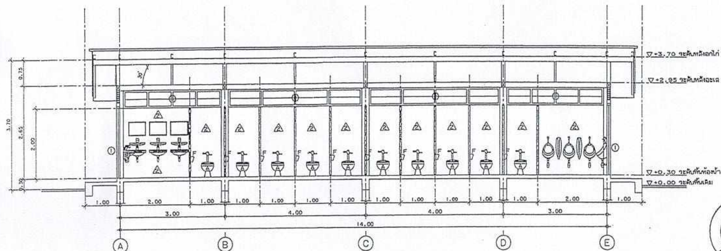
รูปตัด ๘ ห้องน้ำชาย ๖๓๖๖๖ 1:50 (แบบปรับปรุงรายการที่ 10)
