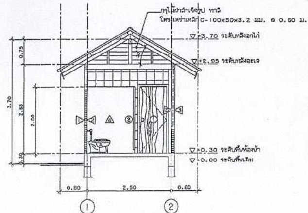
รูปตัด A ห้องน้ำหญิง มาตราส่วน 1:50 แบบปรับปรุงรายการที่ (11)
