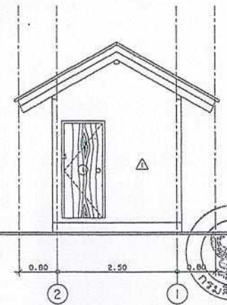
รูปด้านขวาห้องน้ำชาย มาตราส่วน 1:50 (แบบรับปรุงรายการที่ 10)
