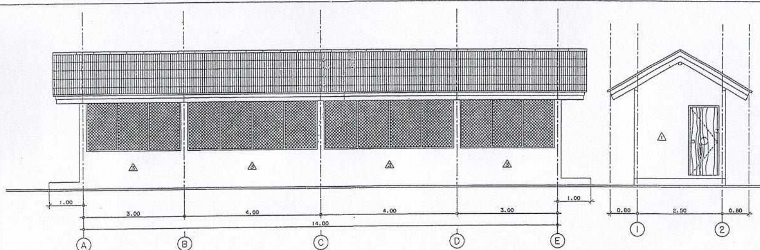
รูปด้านหน้าห้องน้ำหญิง ภาคเช้า 1:50 (แบบปรับปรุงรายการที่ 11)
