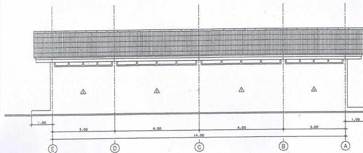
รูปด้านหลังห้องน้ำชาย มาตราส่วน 1:50 (แบบรับปรุงรายการที่ 10)
