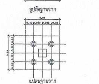
แปลนขยายฐานจาก F1 มาตราส่วน 1:25
