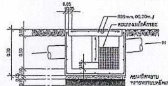
รูปตัดขยายบ่อดักขยะ-ไขมัน คสล. ขนาดฐาน 1 : 25
