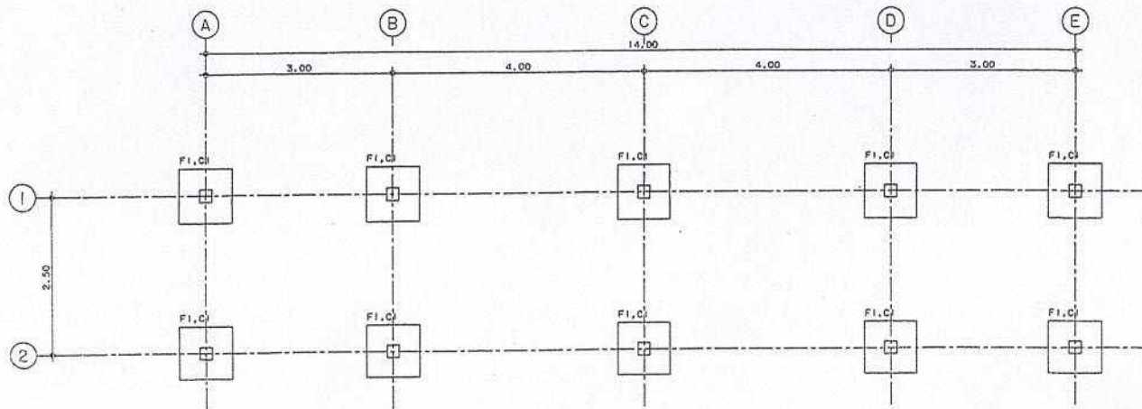
แปลนฐานจากห้องน้ำชาย มาตราส่วน 1:50 (แบบรับปฐมาภรณ์ที่ ๑๐)
