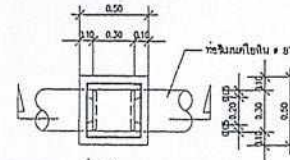
แบบขยายบ่อพัก คสล. (M.H.) ขนาดฐาน 1 : 25
