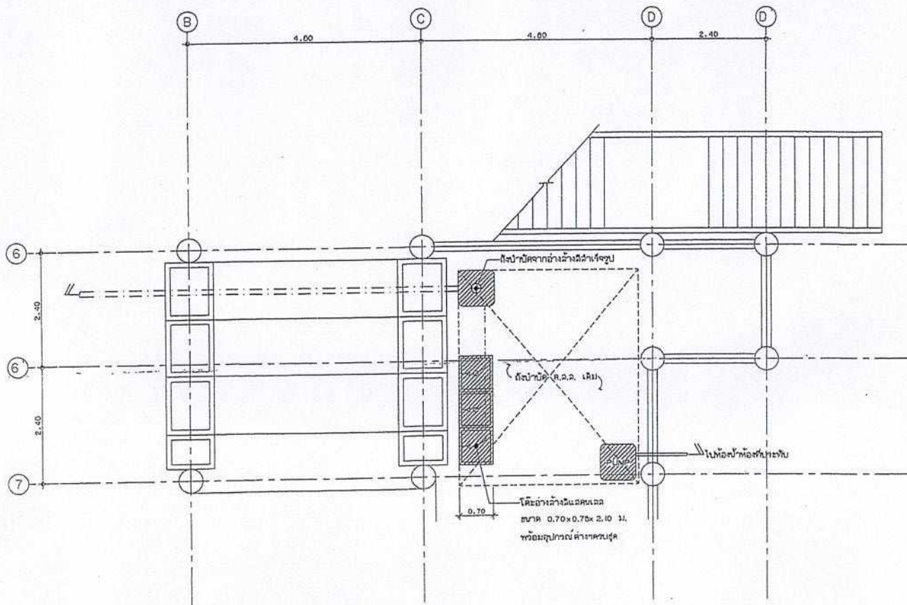
แปลนส่วนที่ล่างลิ (ซ้าย) มาตราส่วน 1:50 แบบรับปรุงรายการที่ (7)
