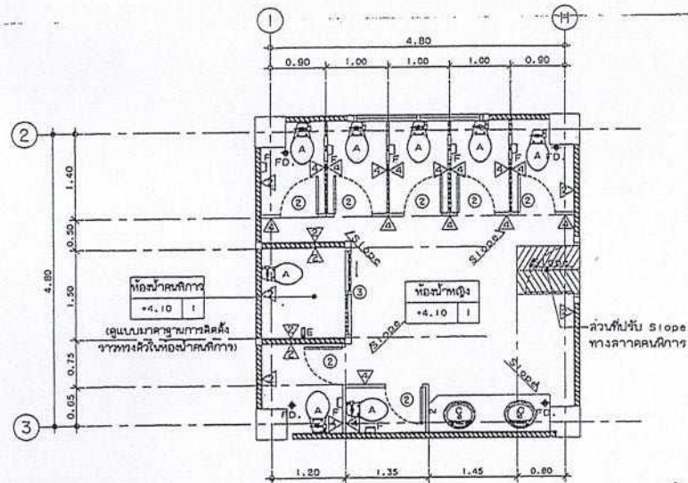
แปลนห้องน้ำดิบ ชั้นที่ 2 มาตราส่วน 1:50 (แบบปรับปรุงรายการที่ 3)
