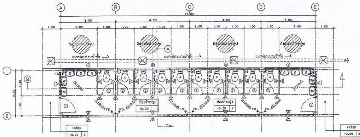
แปลนพื้นที่ห้องน้ำหญิง (ก่อสร้างใหม่นอกอาคาร)
