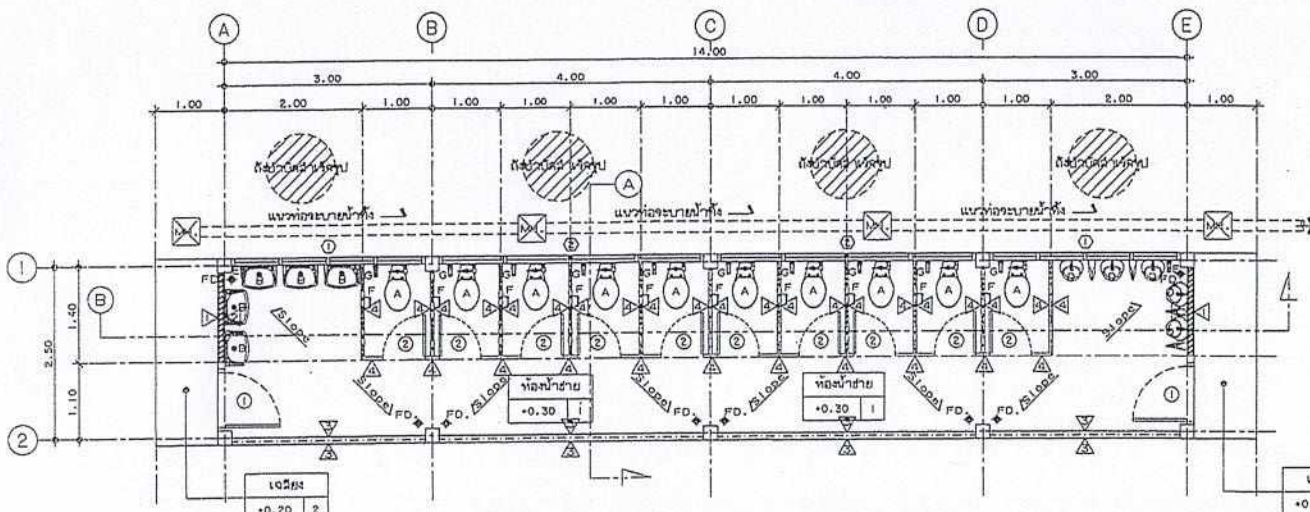
แผนผังห้องน้ำชาย (ก่อสร้างใหม่นอกอาคาร)
