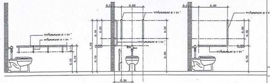
แบบขยายการติดตั้งจาวทรงตัวสำหรับโถชักโครก มาตราส่วน FREE
