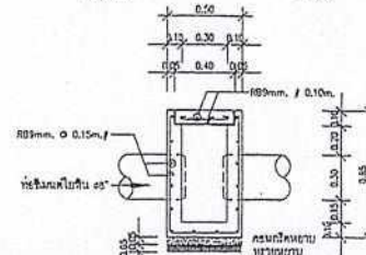
รูปตัดขยายบ่อพัก คสล. ขนาดฐาน 1 : 25
