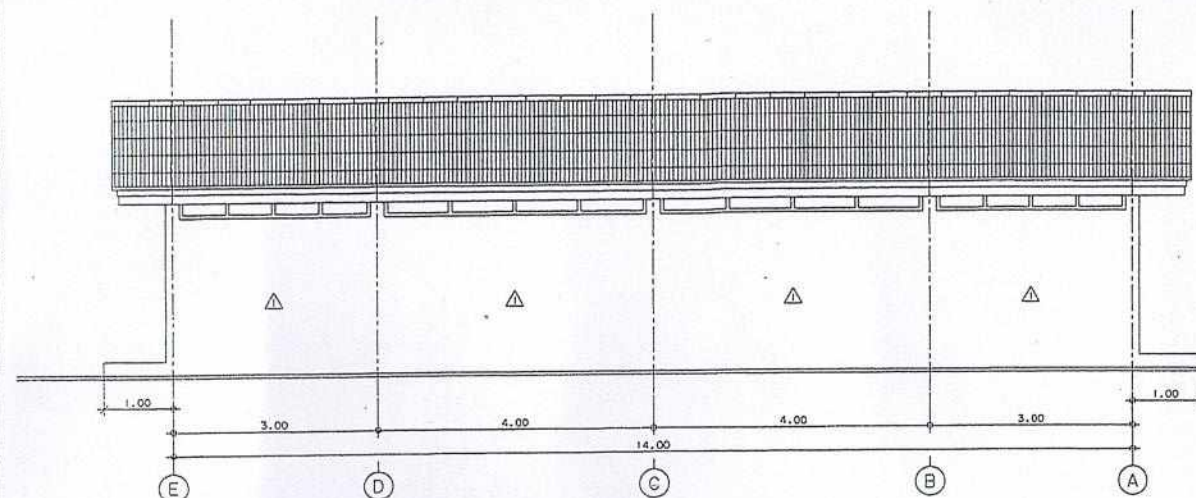
รูปด้านหลังห้องน้ำหญิง ภาคเช้า 1:50 (แบบปรับปรุงรายการที่ (11) )
