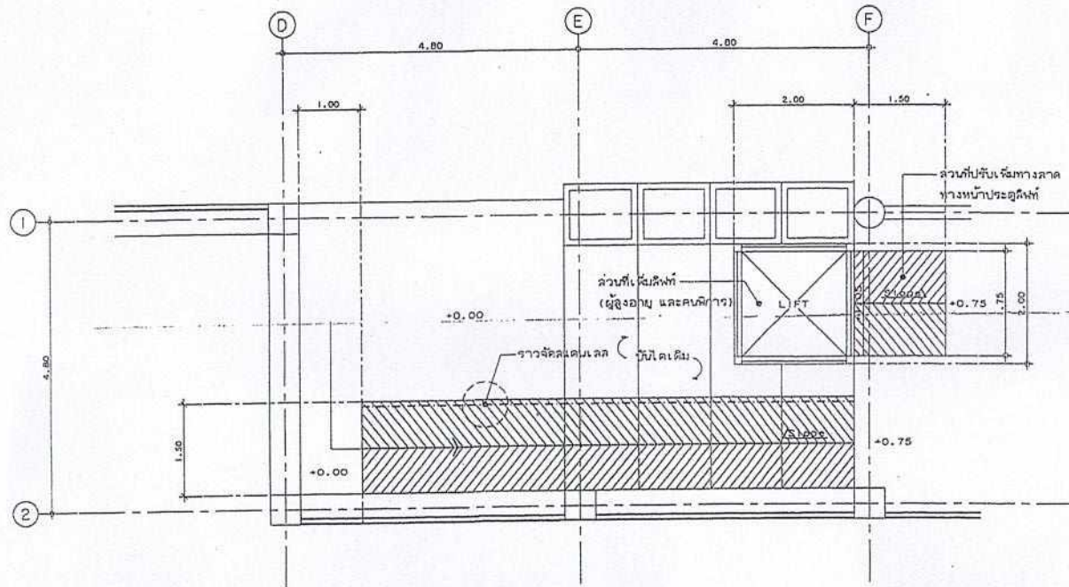
แปลนทางลาด และลิฟท์คนพิการ ภาคส่วน แบบปรับปรุงรายการที่ (๑) 1:50
