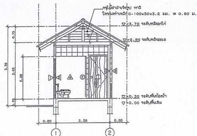
รูปตัด A ห่องน้ำชาย มาตราส่วน 1:50 (แบบปรับปรุงรายการที่ 10)
